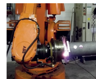
ROBOTERSCHWEIßEN MIG/MAG - Konturschweißen
