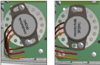
Bild 1: Potiverstellung bis 20°: Verstellung innerhalb der Langlöcher. Schrauben werden nicht versetzt.
