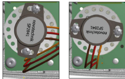
Bild 2: Potiverstellung 20° bis 360°: Schrauben werden versetzt.
