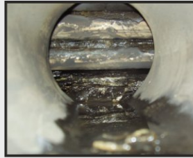
Abgaswärmetauscher, abgas- und wasserseitig
