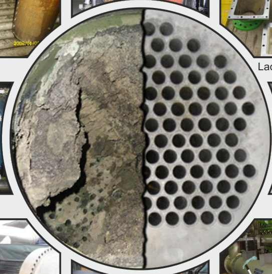
Ladeluftkühler
