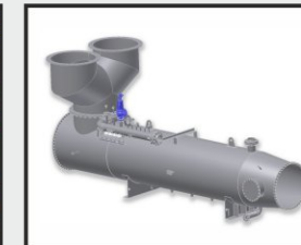
Abgaswärmetauscher Rohrleitungen, Bypass
